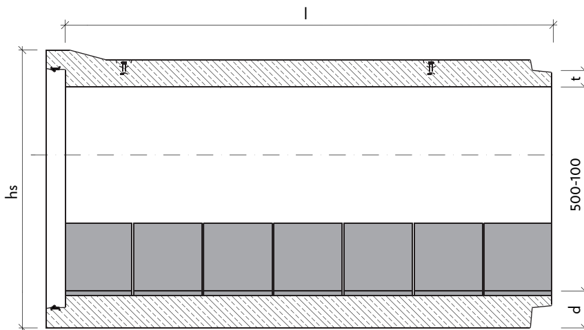
Podélný řez
